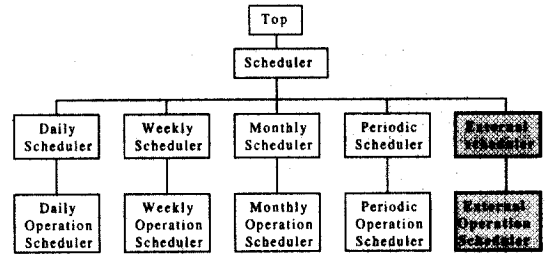
(그림 3) 확장된 Scheduler MO Class 상속 계층구조
