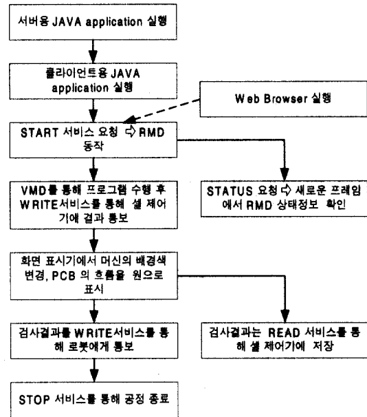
(그림 13) 데모라인의 동작순서
