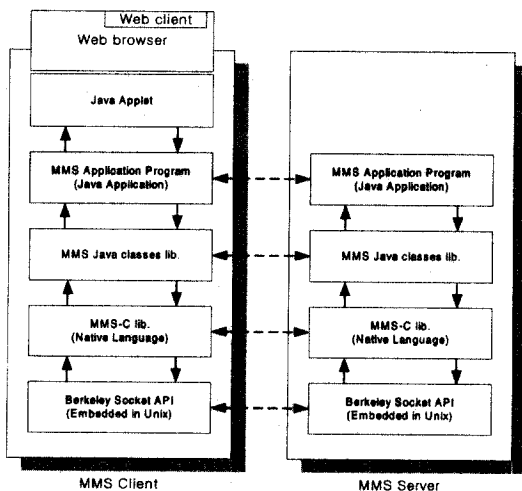
(그림 11) 응용 프로그램의 메시지 전달 구조
