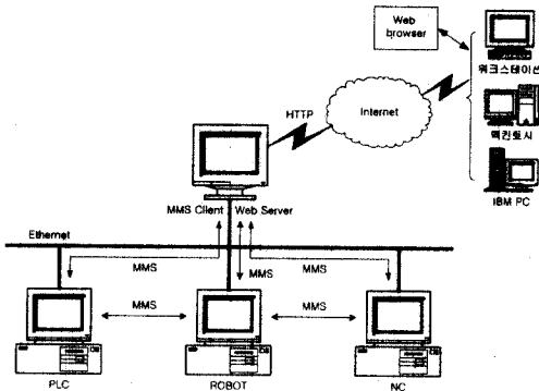
(그림 10) WWW을 통한 MMS 이용 모델
