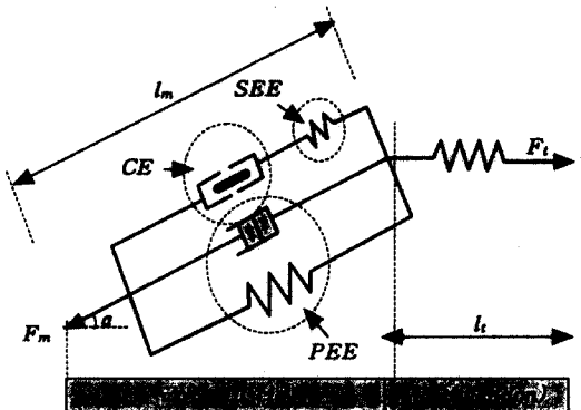
(그림 2) 근육-힘줄구조의 기계요소적 표현[20]( \alpha \neq 0 )
