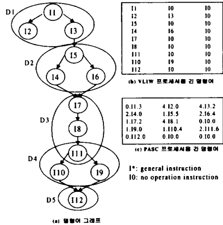
(그림 5) 두 가지 프로세서의 긴 명령어 코드
