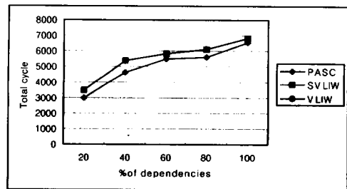
(그림 13) 자료종속성에 따른 총 실행사이클
