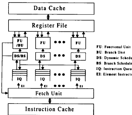
(그림 6) PASC 프로세서 구조
