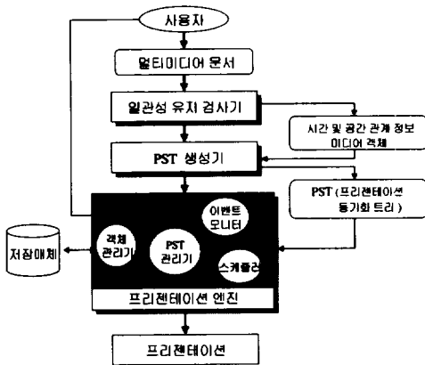
(그림 10) 모델의 구성도 (Fig. 10) Model architecture
