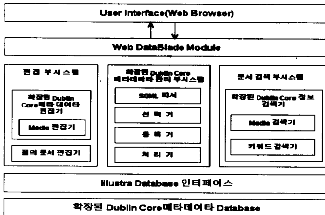
(그림 5) xD-MMS의 구조 (Fig. 5) Architecture of xD-MMS
